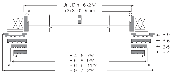
Double Door Unit
